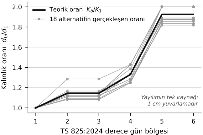
Şekil 2. Gerekli kalınlığın bölgeler arası oranı
